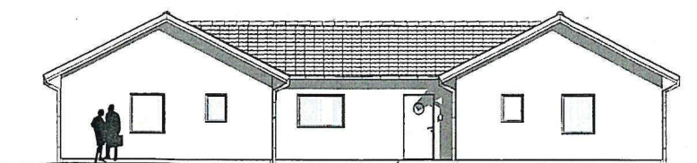
FASAD MOT SYDVÄST 1:100
