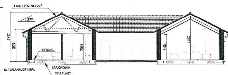
SEKTION B-B 1:100
