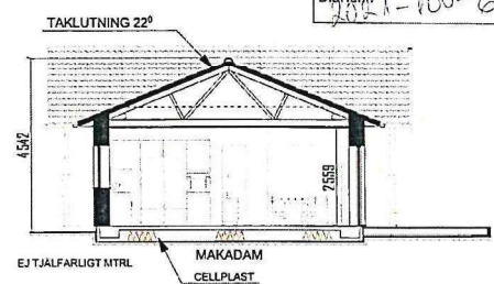
SEKTION A-A 1:100
