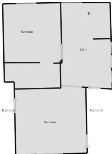
Planritning, övervåning. Ej skalenlig, avvikelser förekommer
